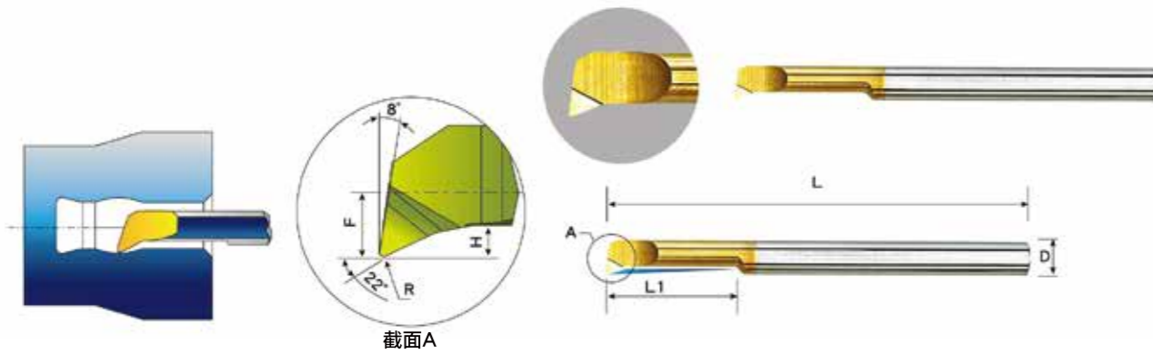
MPR 微型車刀 Micro Turning Cutter
